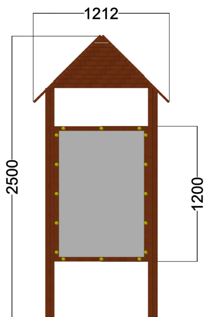
Dimensiones generales
