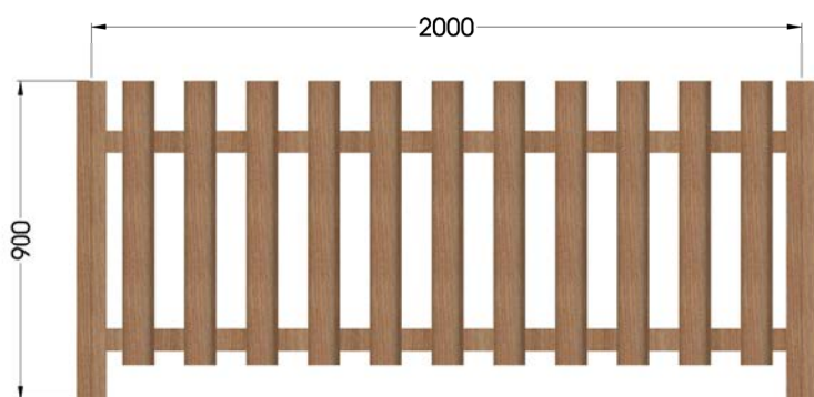
Dimensiones generales
