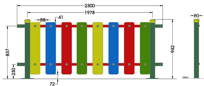
Dimensiones generales
