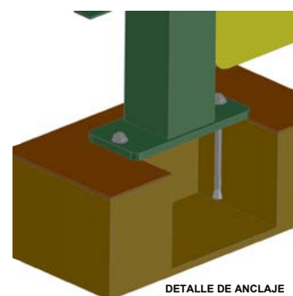
Cimentación
