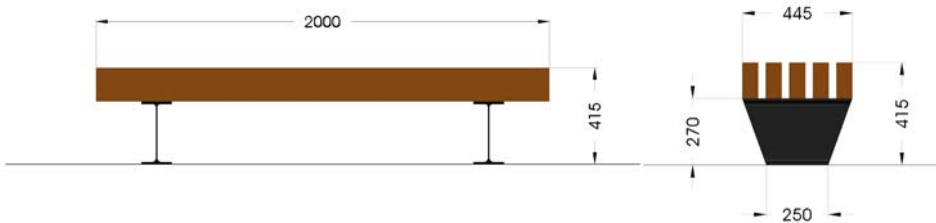
Dimensiones generales
