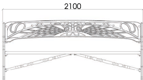
Dimensiones generales
