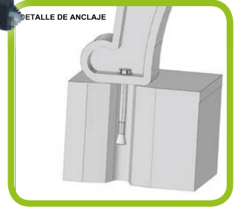
Cimentación
