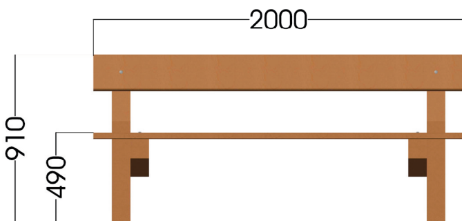
Dimensiones generales
