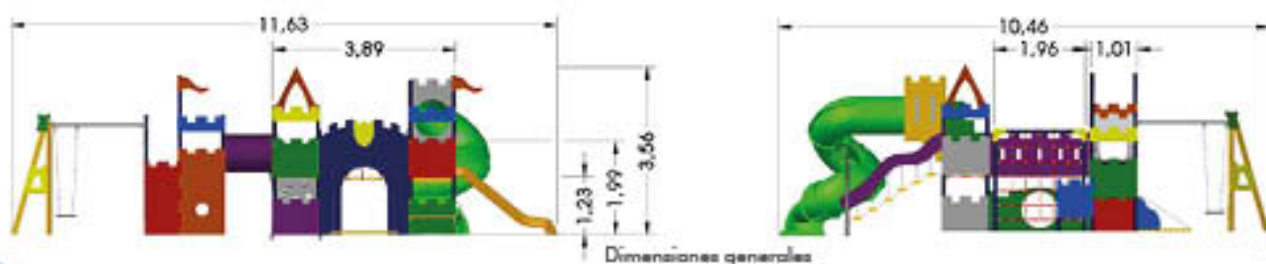
Dimensiones generales
