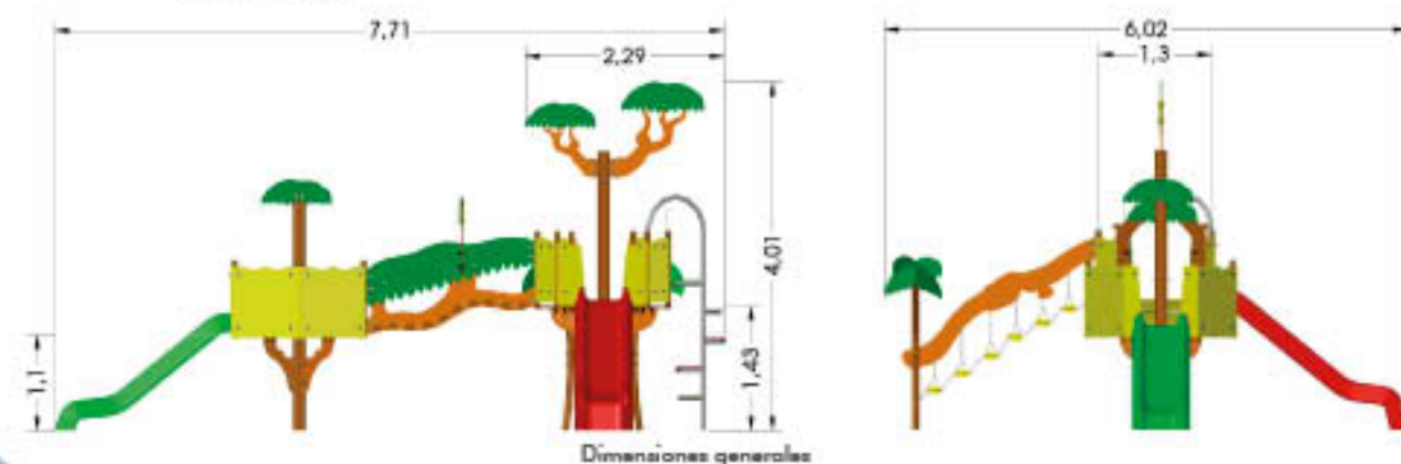
Dimensiones generales
