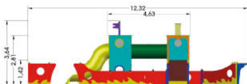
Dimensiones generales
