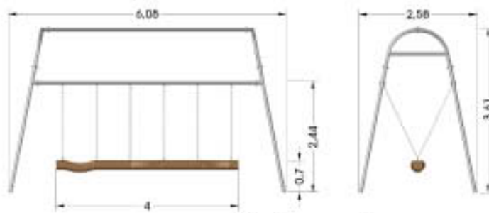
Dimensiones generales
