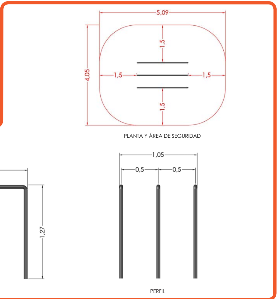
Dimensiones generales
