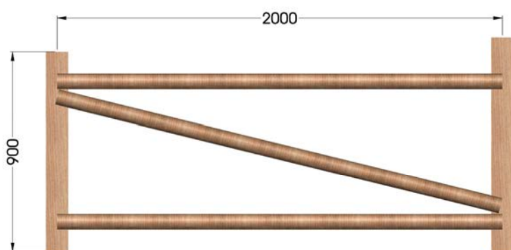
Dimensiones generales
