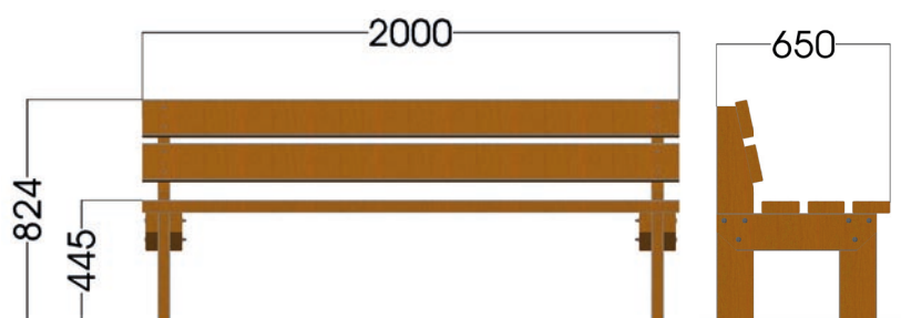
Dimensiones generales
