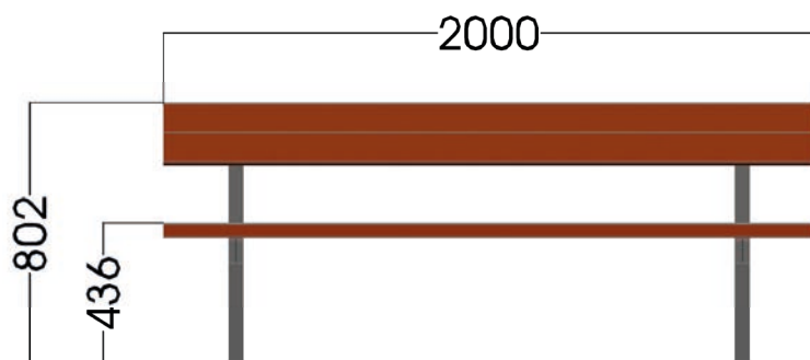
Dimensiones generales
