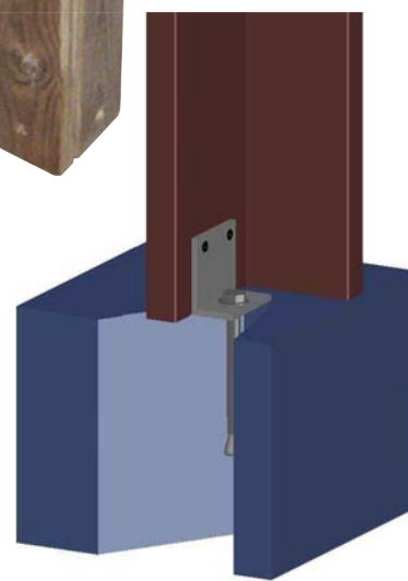
Cimentación
