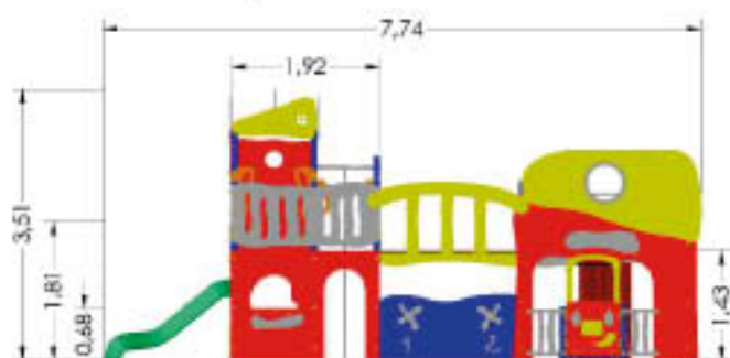
Dimensiones generales
