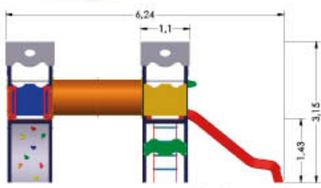
Dimensiones generales
