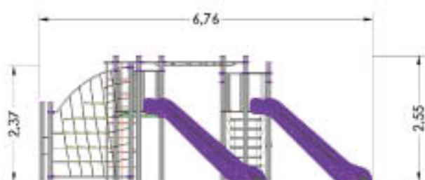
Dimensiones generales
