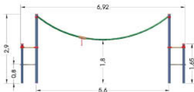
Dimensiones generales
