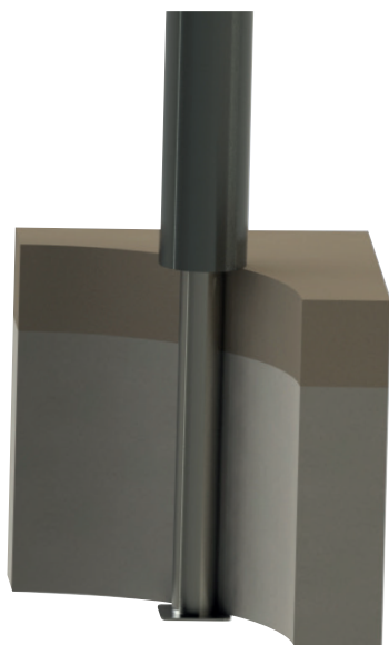
Anclaje para suelo blando de tubo metálico galvanizado enterrado en dado de hormigón de 400x400x500mm cubierto de arena.
